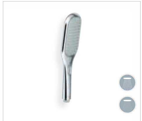
27 274 000 1 2 3 4 5 Chuveiro de mão, jactos: Rain, Smart Rain 27 281 000 1 2 3 4 5 Com limitador ecológico de caudal 9.4 l/ min
